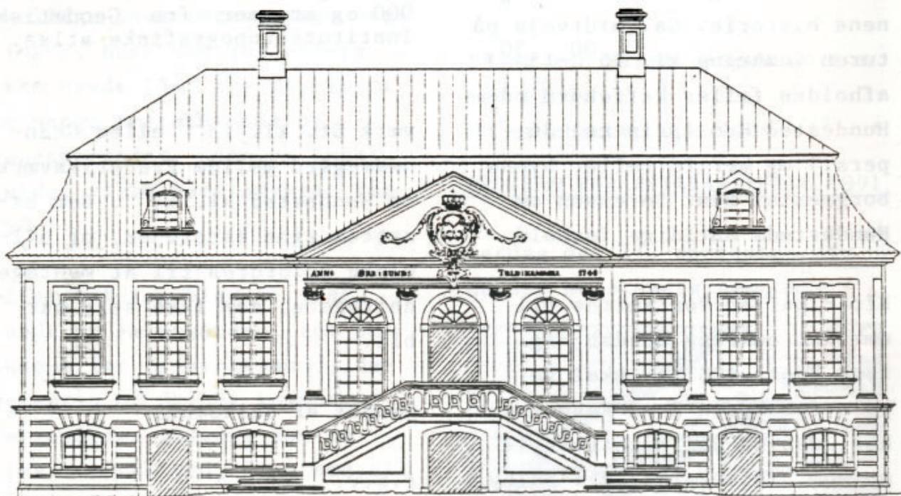
Øresunds Toldkammer tegnet af murmester Niels Basse i 1740. Bygningen stod færdig 1742. Rekonstruktion tegnet af Lars Bjørn Madsen.
