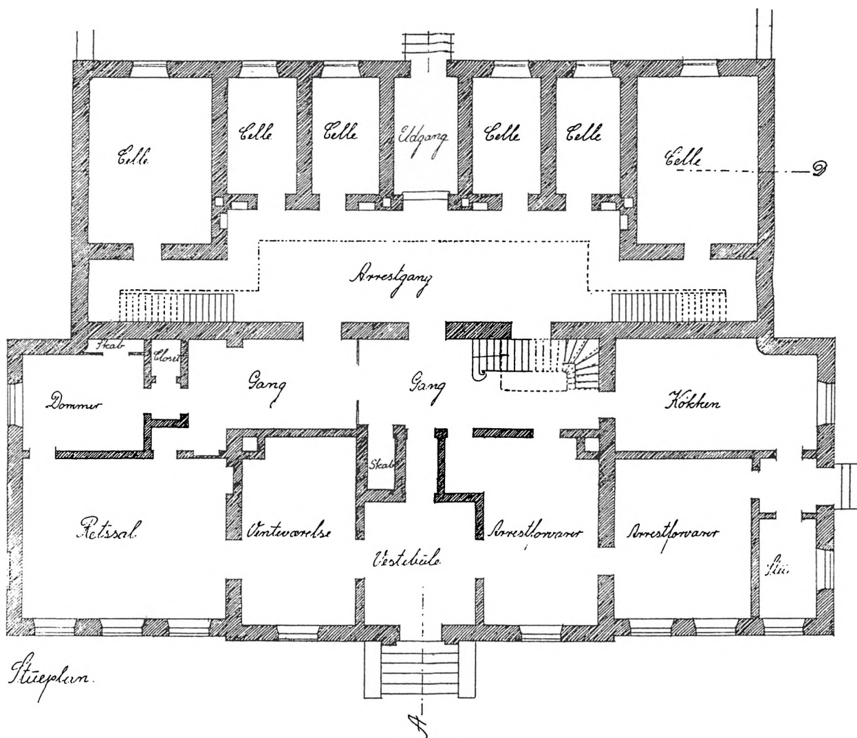
Arkitekttegning fra 1931 af stueetagen af ting- og arresthuset, Kronborg østre Birk. (Fredensborg-Humblebæk Lokalhistoriske Arkiv)
